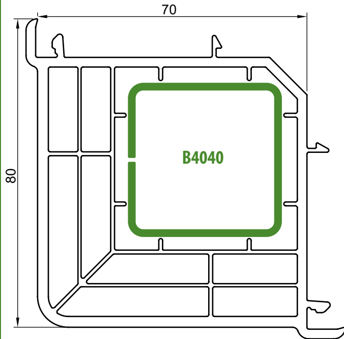
Łącznik 90° 57063
